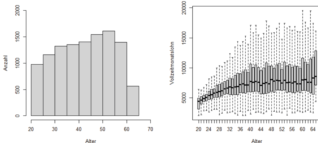
Histogramm und Boxplot (ohne Ausreisser) zum Merkmal Alter
